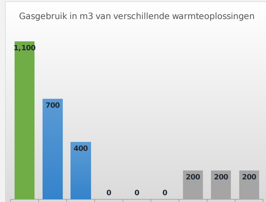
Figuur 2. Gasvraag diverse warmteoplossingen voor een rijwoning met basisniveauisolatie (65 kWh/m 2 )
