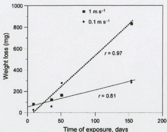
Figuur 2.5 Massa afname van vislode in de Zweedse "Adran brook" gedurende 160 dagen, bij verschillende doorstroomsnelheden (uit: Jacks et al. 2001).
