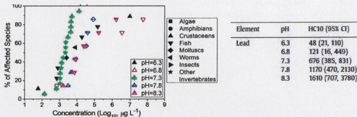
Figuur 2.7 Acute effectconcentraties van opgelost lood voor verschillende soorten waterorganismen, geclusterd per pH van het test medium (uit: Wang, Meador et al. 2009) 18 , en afgeleide HC10 waardes. De x-as geeft de logaritmische concentratie in µg/L. Y-as geeft de cumulatieve fractie van soorten weer ten opzichte van het totale aantal soorten per dataset.
