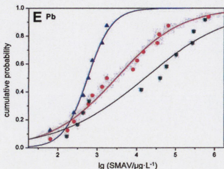
Figuur 2.8 Acute effectconcentraties van opgelost lood voor verschillende types waterorganismen: watervlooiën (blauwe driehoek), andere invertebraten (rode cirkel), en vissen (groene vierkant) (uit: Xin et al. 2015) 19 . De x-as geeft de logaritmische concentratie in µg/L. Y-as geeft de cumulatieve fractie van soorten weer ten opzichte van het totale aantal soorten per dataset.
